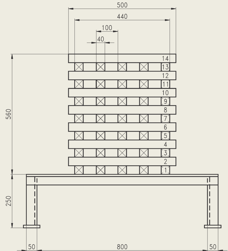
Vista frontale (identica per tutti i focolari)
